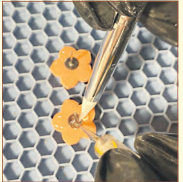
Nach dem Ablösen vom Fliesenuntergrund werden die Teile mit einem feinen Schleifbohrer entgratet. Anschließend legt Janina Wegner die Vorderteile der Ohrhinge auf ein Silikonpad, beträufelt diese mit UV-Resin-Kleber und fixiert mittig die Edelstahlstecker.
